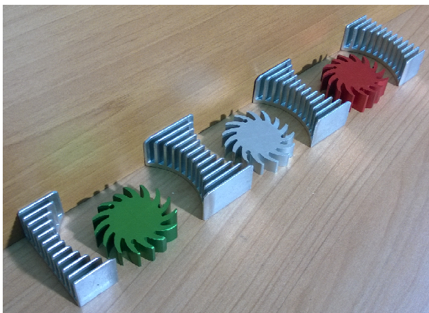
BAR MILLING DIAMETRO: da 27mm a 50/52mm
